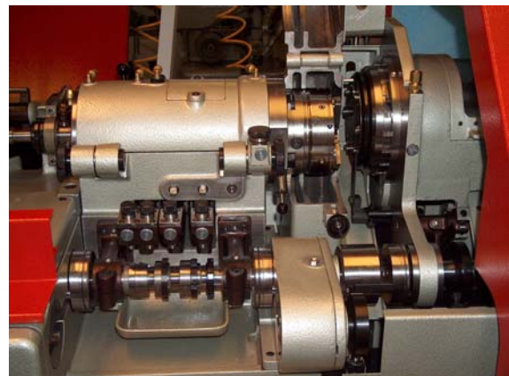
Mandrin Rotatif à 7'100 t/min. et revolver à 4 positions..
